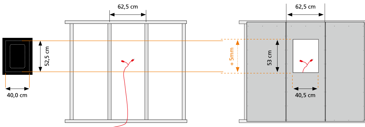
1. UNTERKONSTRUKTION Standard CW-Profil im Abstand von 62,5 cm, Verkabelung planen und legen.
