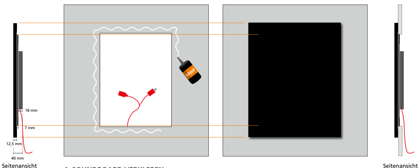
4. SOUNDBOARD VERKLEBEN MWP Montagekleber um den Ausschnitt der Rigipsplatte herum auftragen.
